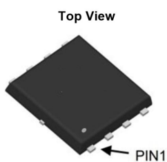
PDFN5x6-8L
